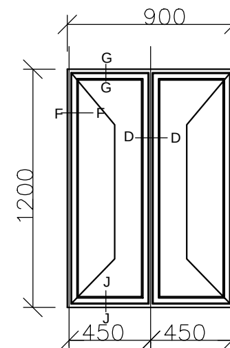
WINDOW TYPE W4
